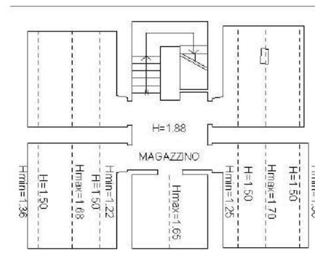
PIANO PRIMO SOTTOSTRADA
