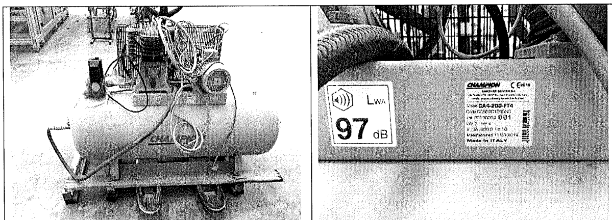
Figura 77 – Compressore per aria compressa CHAMPION CA4-200-FT4
