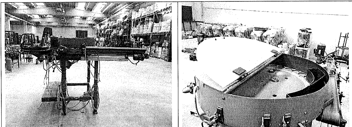
Figura 76 – Macchina O.C.M.G. s.a.s. per caricatore elementi cilindrici
