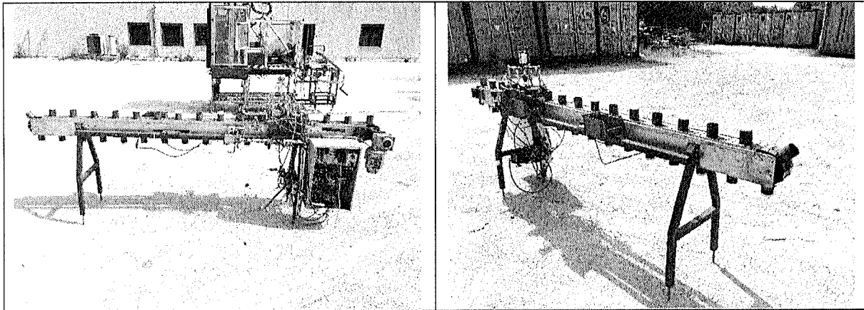
Figura 85 – Macchina per candele elettriche
