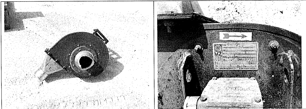
Figura 88 – Aspiratore marca MZ Aspiratori tipo RM 310
