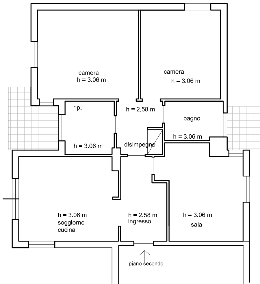
Planimetria appartamento sub. 21 scala 1:100
