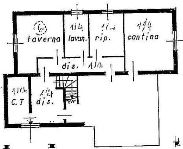
PIANTA SCANTINATO
