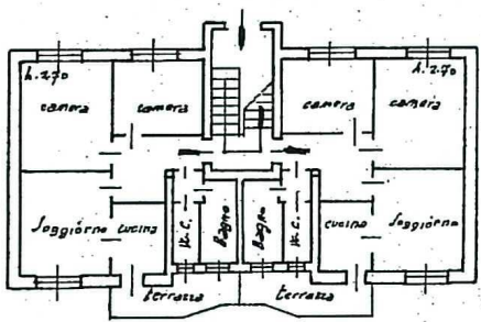
PIANTA PIANO RIALZATO
