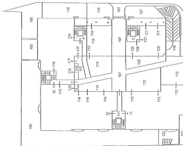
PIANO TERRA E SCOPERTO
