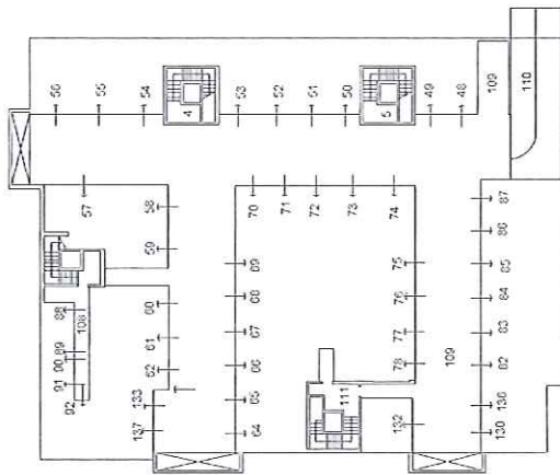
PIANO PRIMO SOTTOSTRADA
