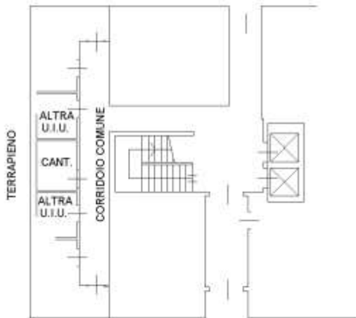
PIANO PRIMO INTERRATO H=2.70
