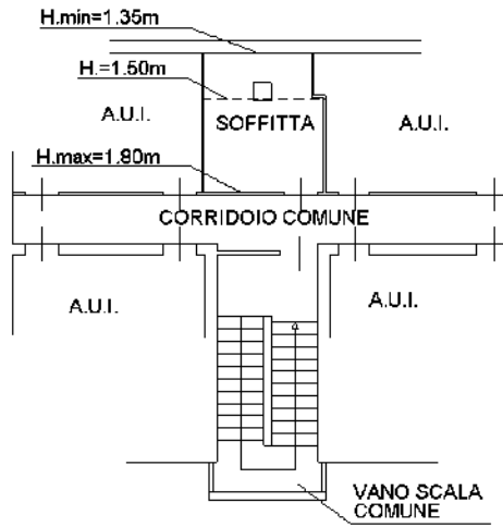
PIANTA PIANO QUARTO(SOTTOTETTO)
