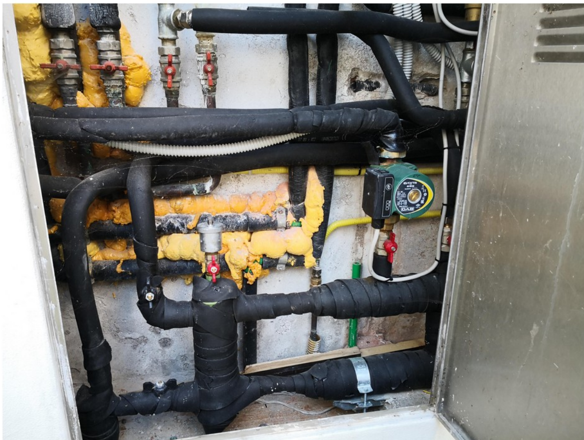
67 - impianto idro termo sanitario distribuzione
