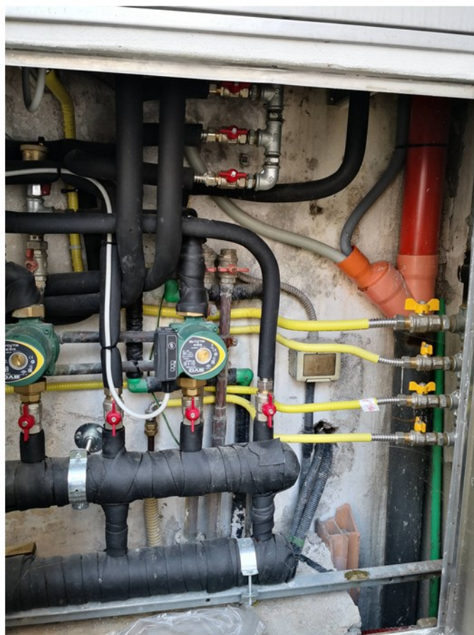
68 - impianto idro termo sanitario distribuzione
