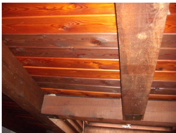
PARTICOLARE DELLA COPERTURA SOTTOTETTO
