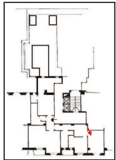
Camera matrimoniale
