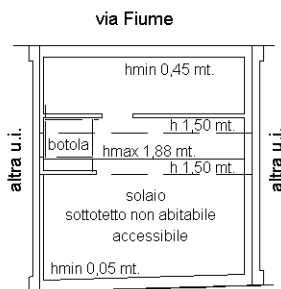
PIANO PRIMO (SOPPALCO)
