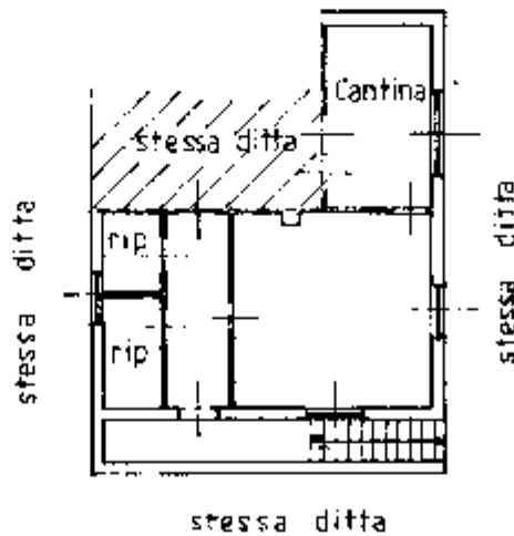
PIANTA P SEMINTERRATO
