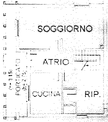
PIANTA PIANO TERRA (H= 2.80)
