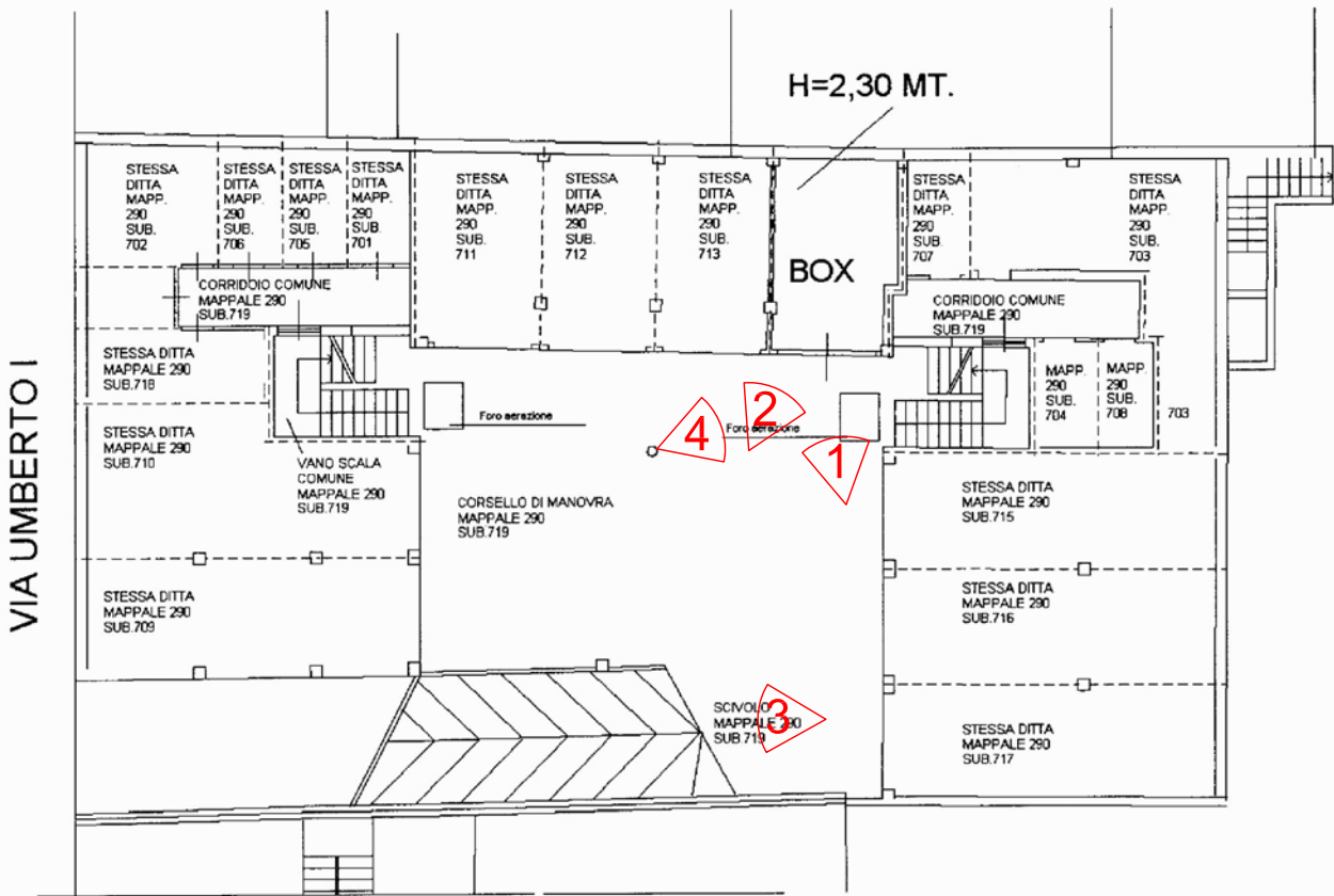
PIANTA PIANO SEMINTERRATO
