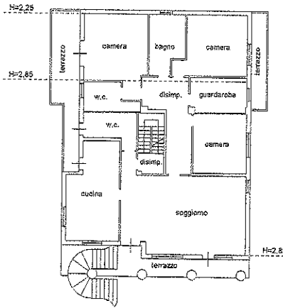
PIANO PRIMO H = 2,85
