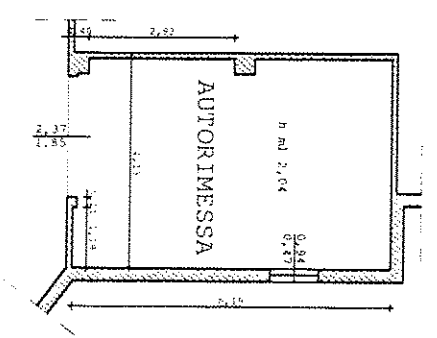
SCHEMA RILIEVO PIANO INTERRATO Scala 1:100
