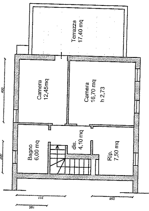
Piano primo
