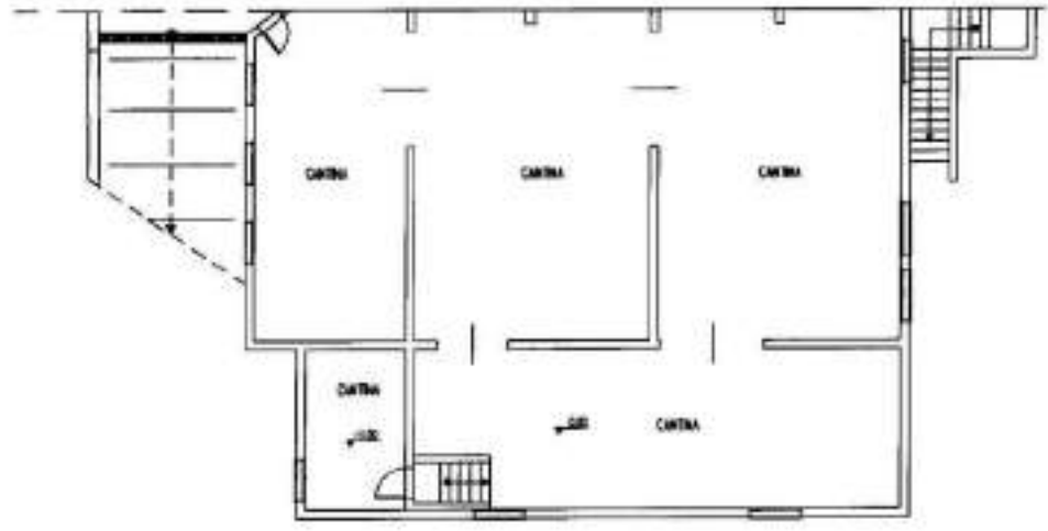
PIANTA PIANO INTERRATO SCALA 1:100 R. 250
