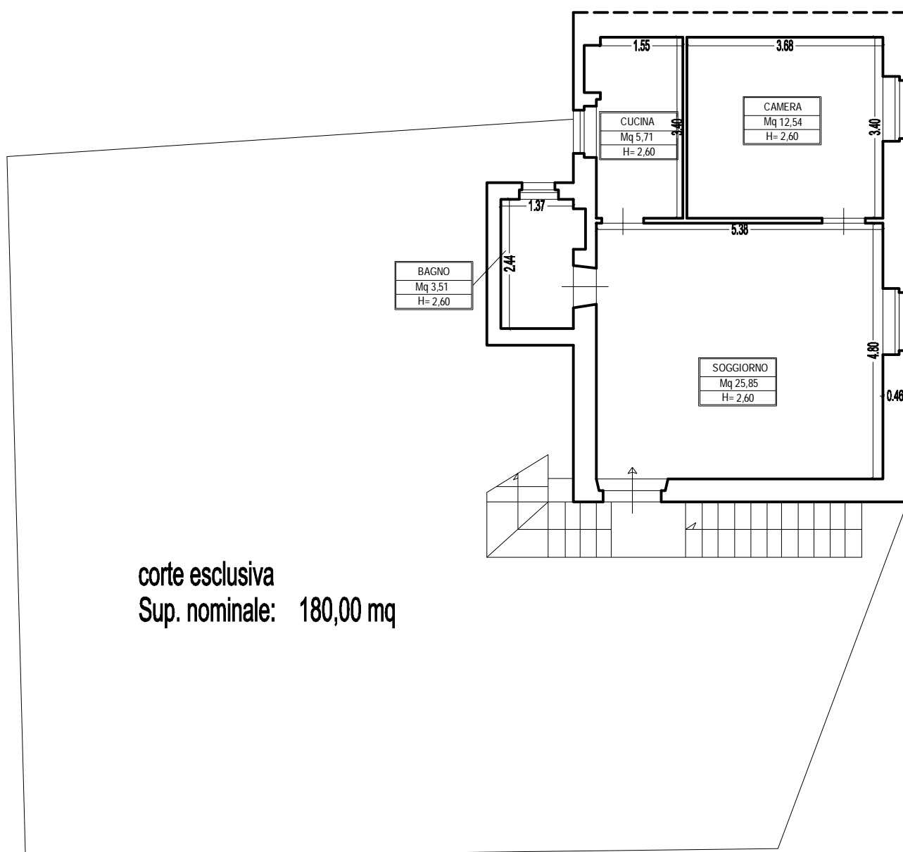
PLANIMETRIA LIVELLO PRIMO scala 1:100
