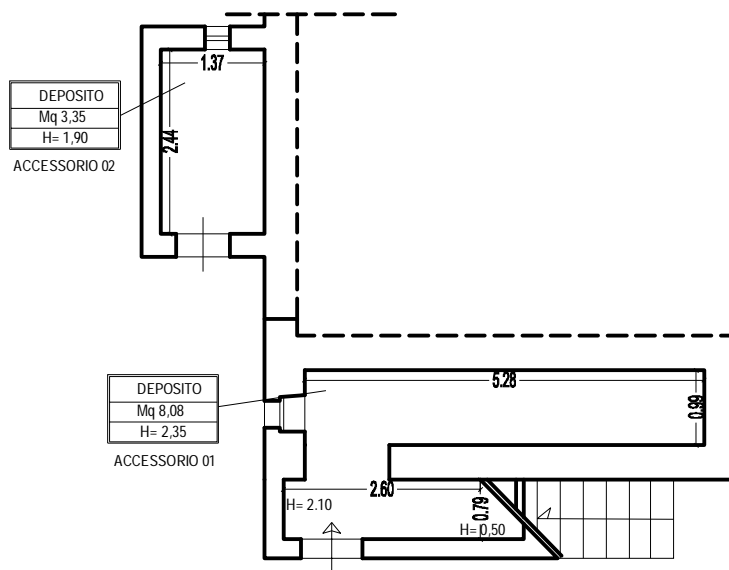
PLANIMETRIA LIVELLO TERRA - ACCESSORI scala 1:100
