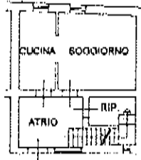
PIANO TERRA. H=cm.248
