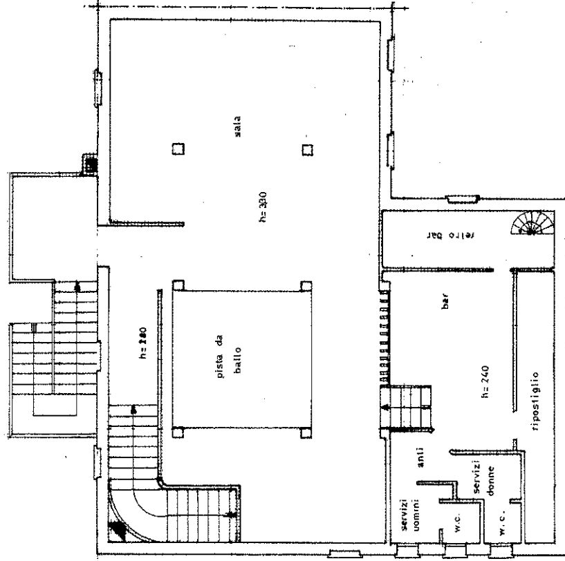
PIANO PRIMO
