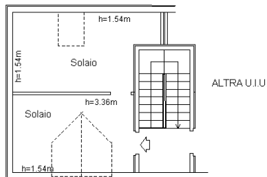
Pianta Piano Terzo
