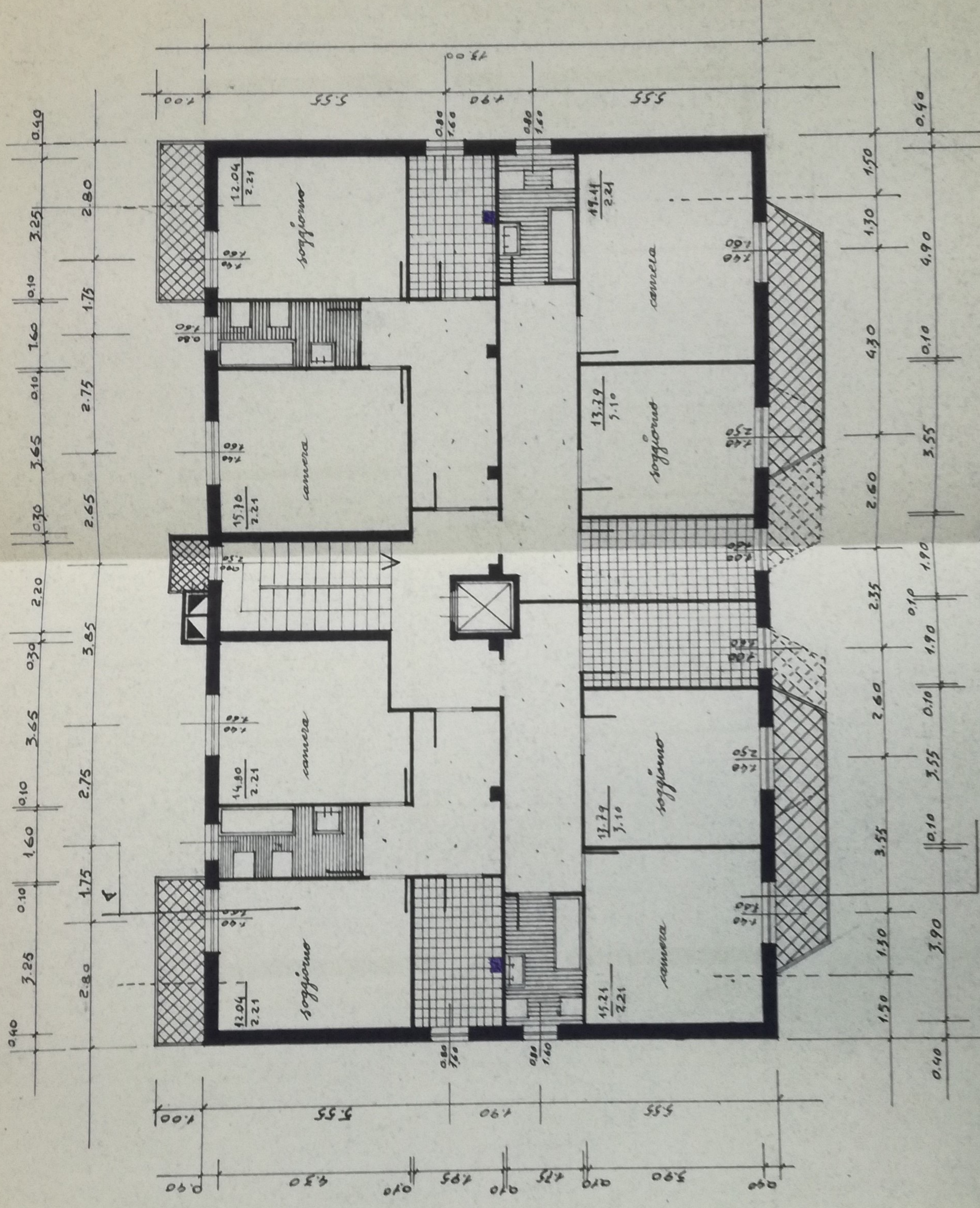
PIANTA PIANO TIPO
