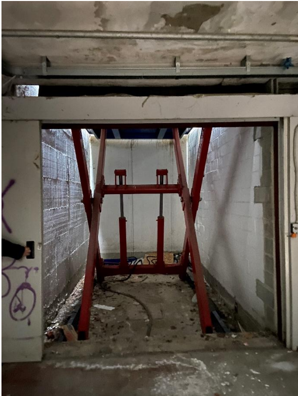
Viste accesso meccanico al piano box
