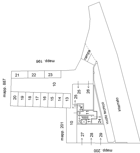
PIANO PRIMO SOTTOSTRADA
