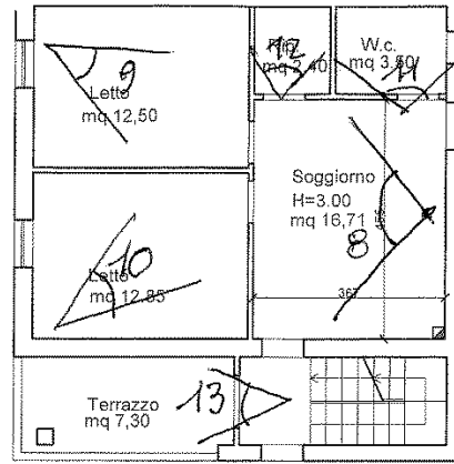
PIANO PRIMO
