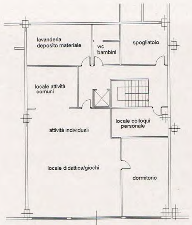
PIANO SOPPALCO H. 2,70
