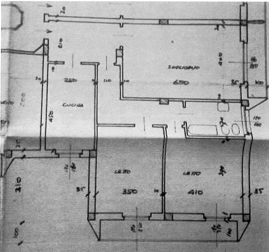
Stralcio della planimetria facente parte del progetto originario.
