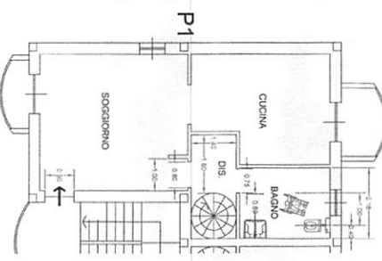
Visibilità appartamenti n.7 e 8 - 1:50
