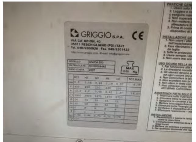
[96] Sezionatrice GRIGGIO UNICA 500_LD.JPG
