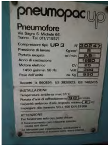
[41] Compressore PNEUMOPAC UP TIPO U3_aLD.JPG
