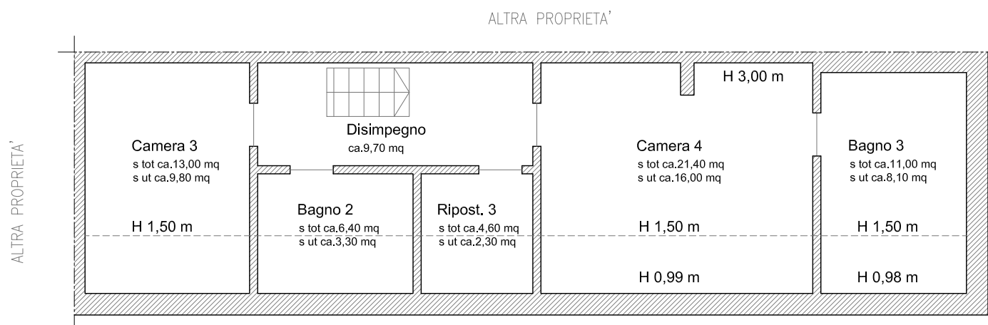
PLANIMETRIA APPARTAMENTO - P 4° Scala 1:200
