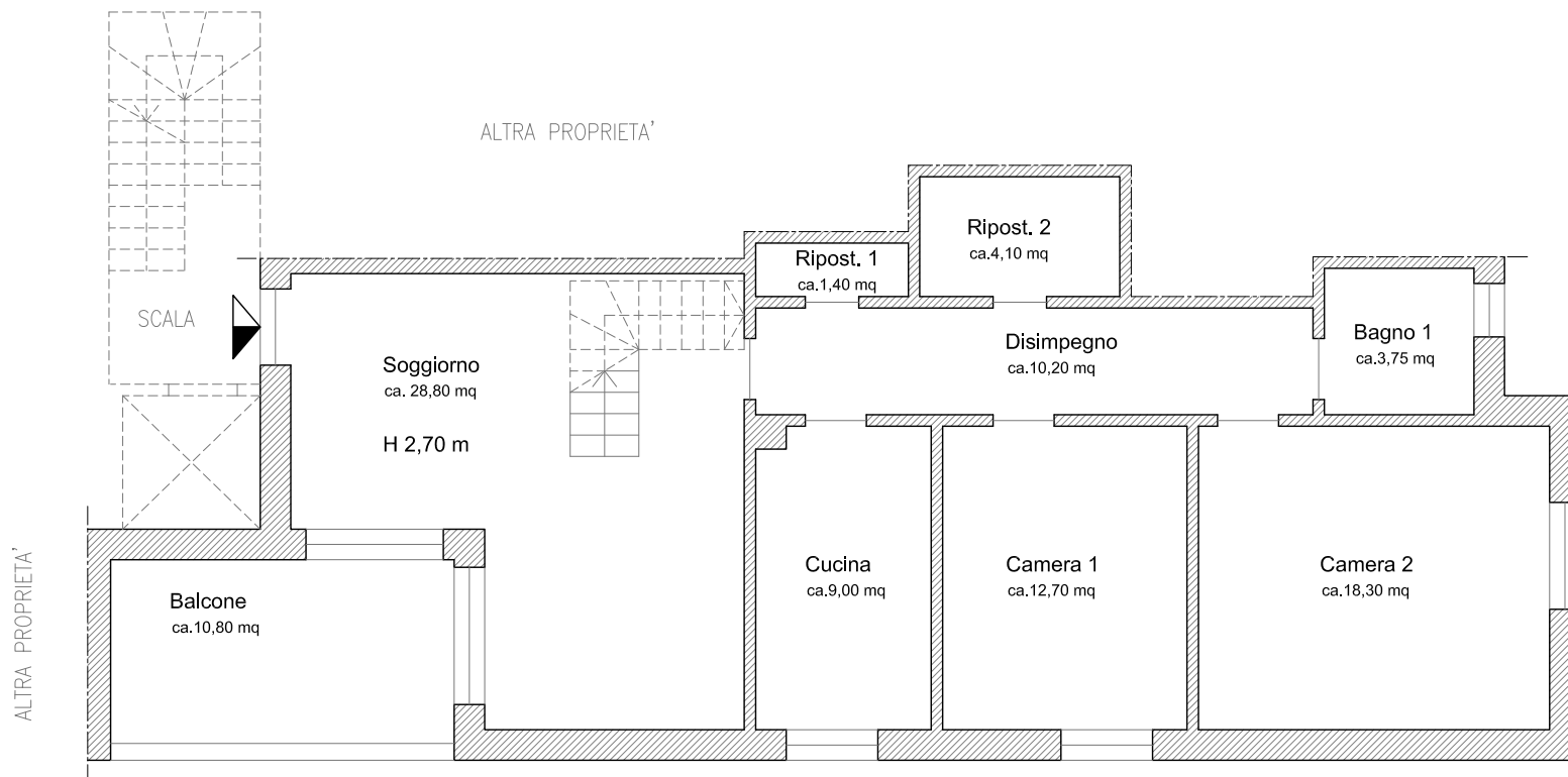
PLANIMETRIA APPARTAMENTO - P 3° Scala 1:200
